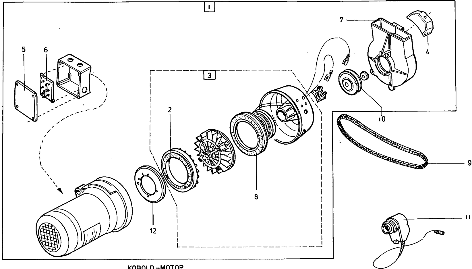
KOBOLD-MOTOR bis 1997
